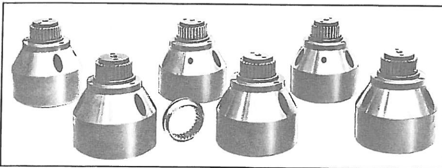
Spanndornsatz für Mehrspindel-Drehautomat
