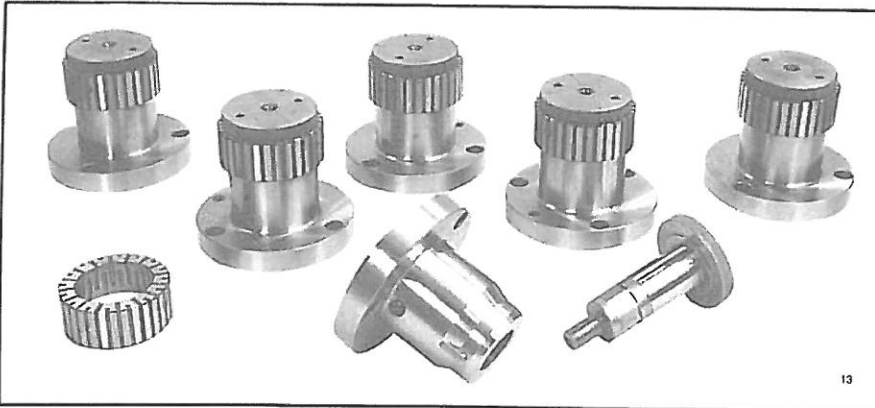
Spanndornsatz für Mehrspindel-Drehautomat – verkürzte Spannhülsen
