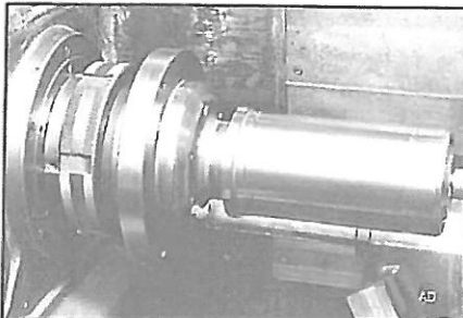
Ausgleichende Doppelspannung mit typischen Werkstücken
