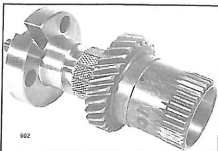
Profilierte Spannhülse zur verbesserten Drehmomentübertragung
