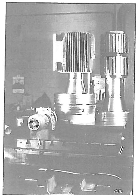
Ausgleichende Doppelspannung/ EM 10 C
