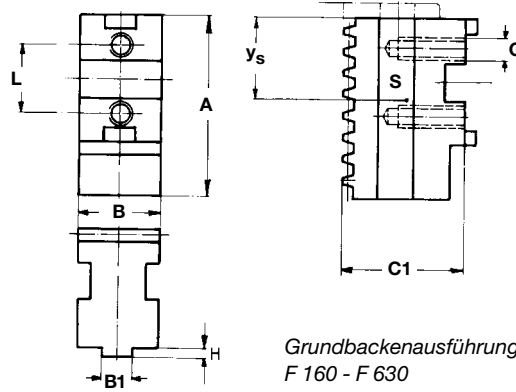
Grundbackenausführung F 125
